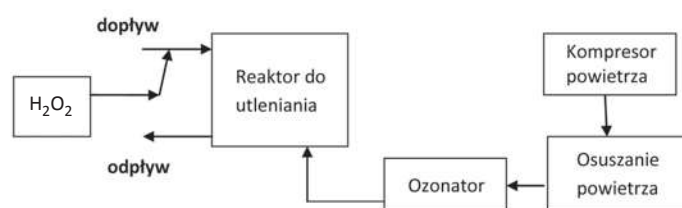
Rys. 1. Schemat procesu Peroxo [Barbusiński 2010]
